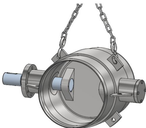
Fig. 4-1: Anhugning i kranøjerne
