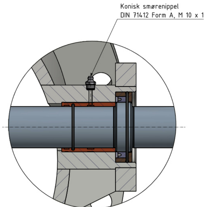
Fig. 7-1: Fedtspærrekammer
