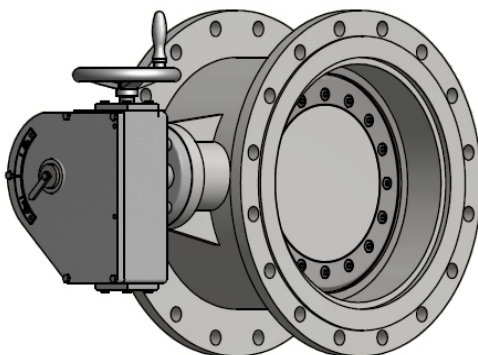
Fig. 5-4: Afspærringsventil med manuel fremdrift ved hjælp af håndhjul
