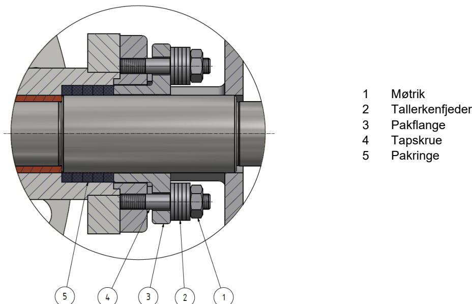
Fig. 7-2: Pakdåse
