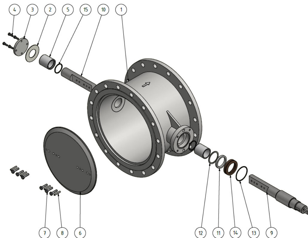
Fig. 3-2: eksempel på en spjældventil
