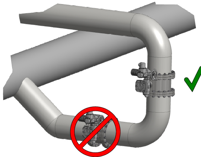
Fig. 5-2: Position i rørledningen/2
