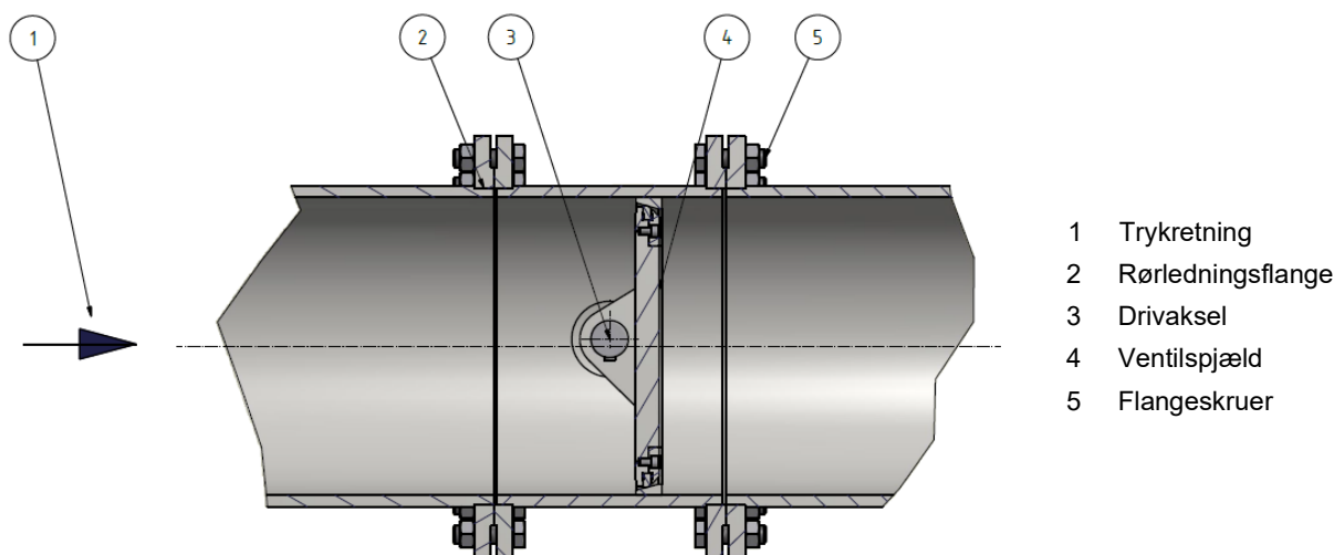
Fig. 5-3: Tværsnit af afspærringsventilen
