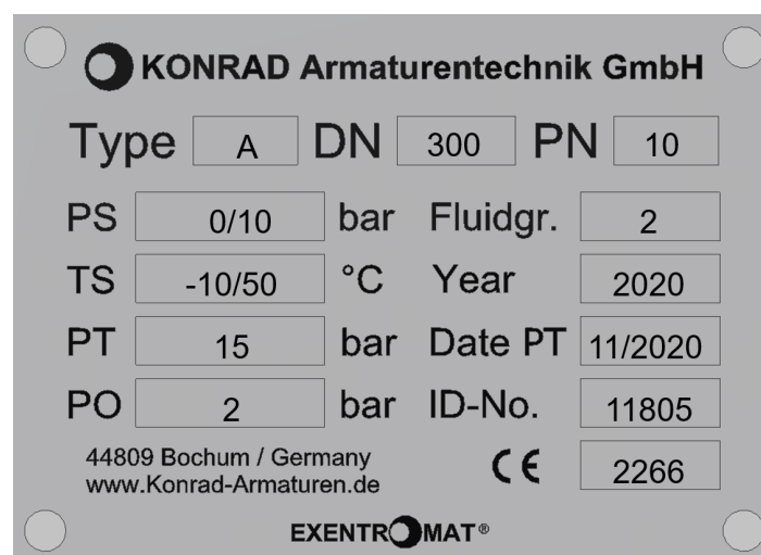
Fig. 3-3: Typeskilt
