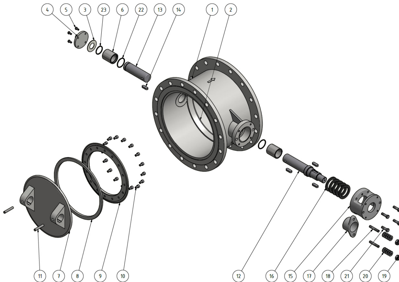
Fig. 3-1: eksempel på en afspærringsventil
