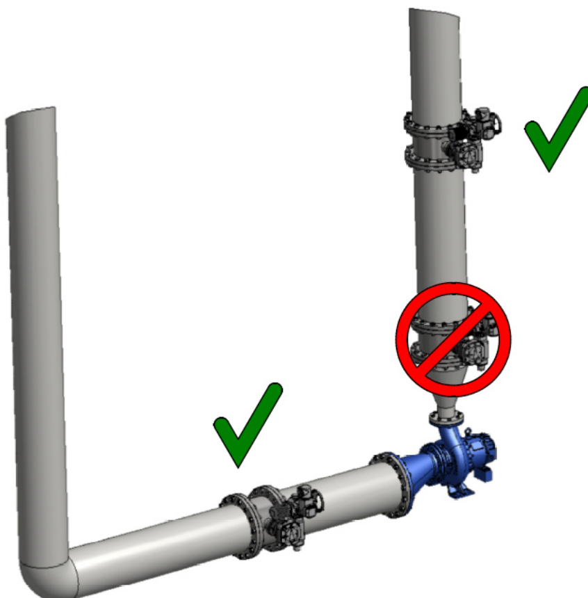
Fig. 5-1: Position i rørledningen/1
