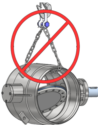
Fig. 4-4: Anhugning gennem armaturhuset
